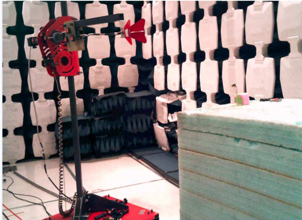
6-18GHz
