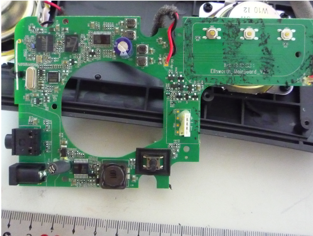
Fig. 5: PCB
