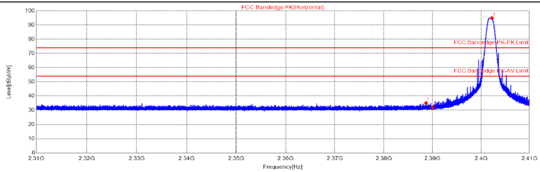
BLE_2402_Ant1/ Horizontal
