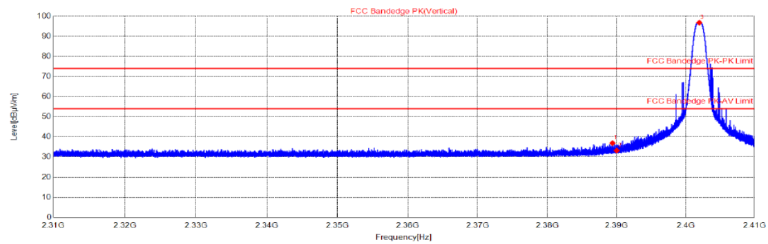
BLE_2402_Ant1/ Vertical
