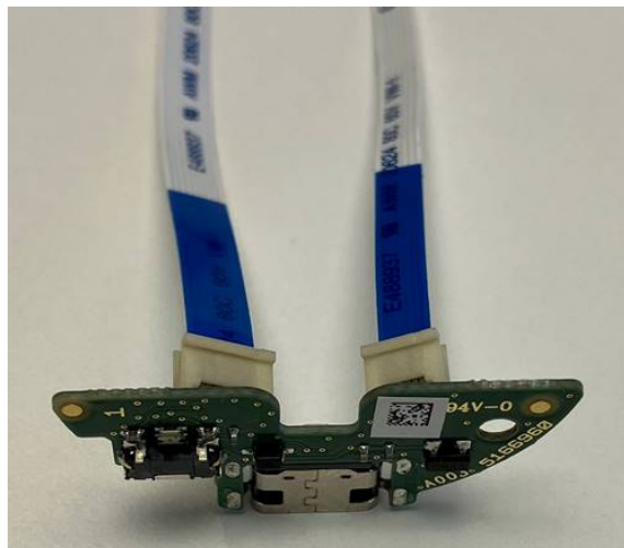
EUT Digital I/O Section
