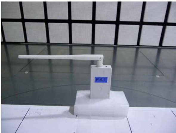
Module:Z-axis / Antenna:X-axis
