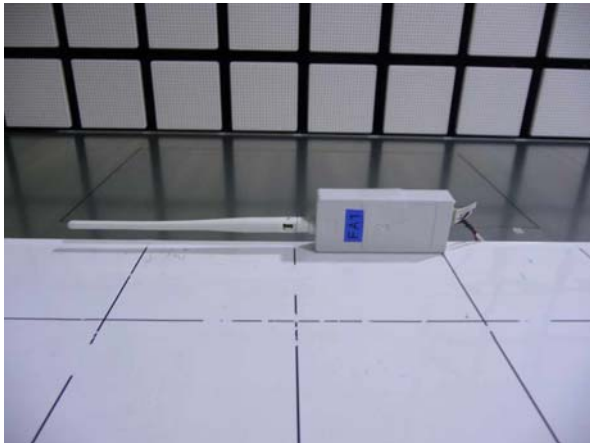
Module:Y-axis / Antenna:X-axis
