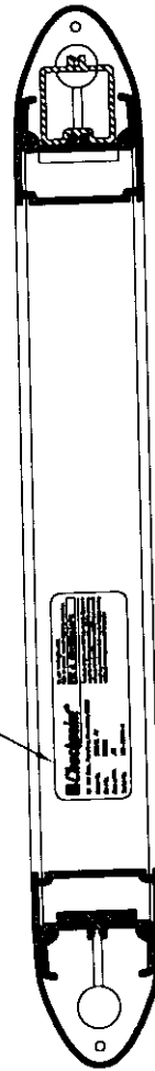
SECTION A--A SCALE: 2/1
