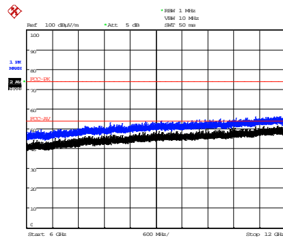
Date: 6.JUL.2016 15:12:27 6 GHz – 12 GHz
