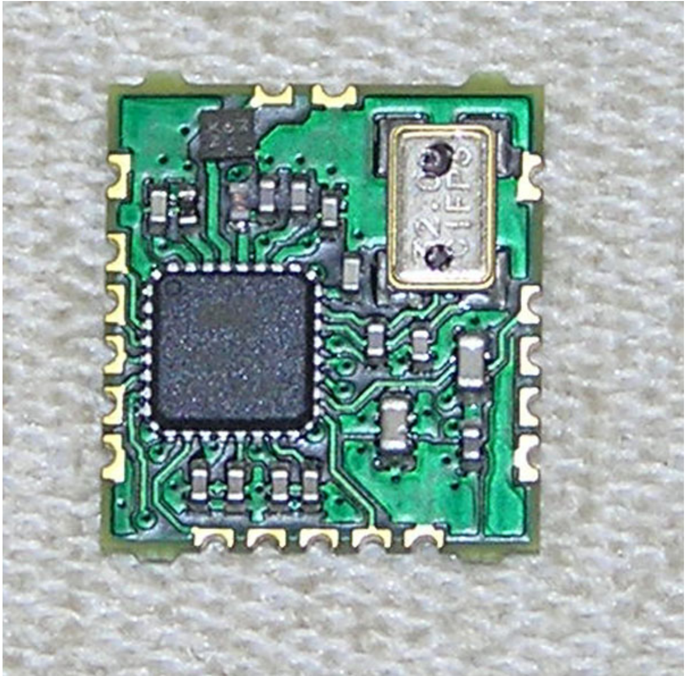
HA18 RF MODULE PCB ZM3102N FRONT
