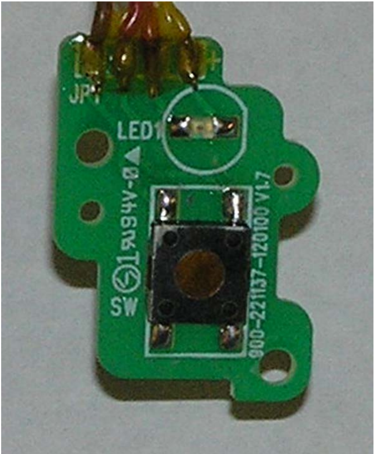
KEYPCB
