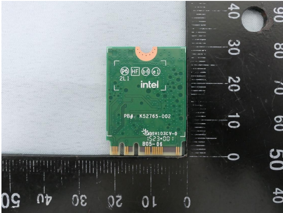
(30) EUT Photo
