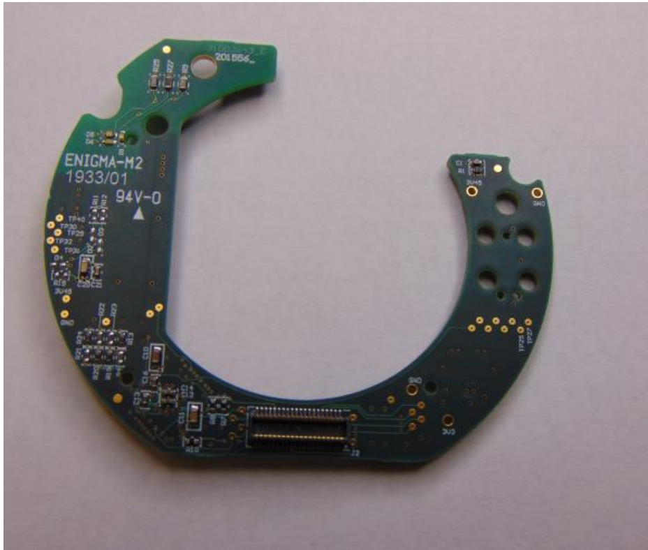
MCU Back
