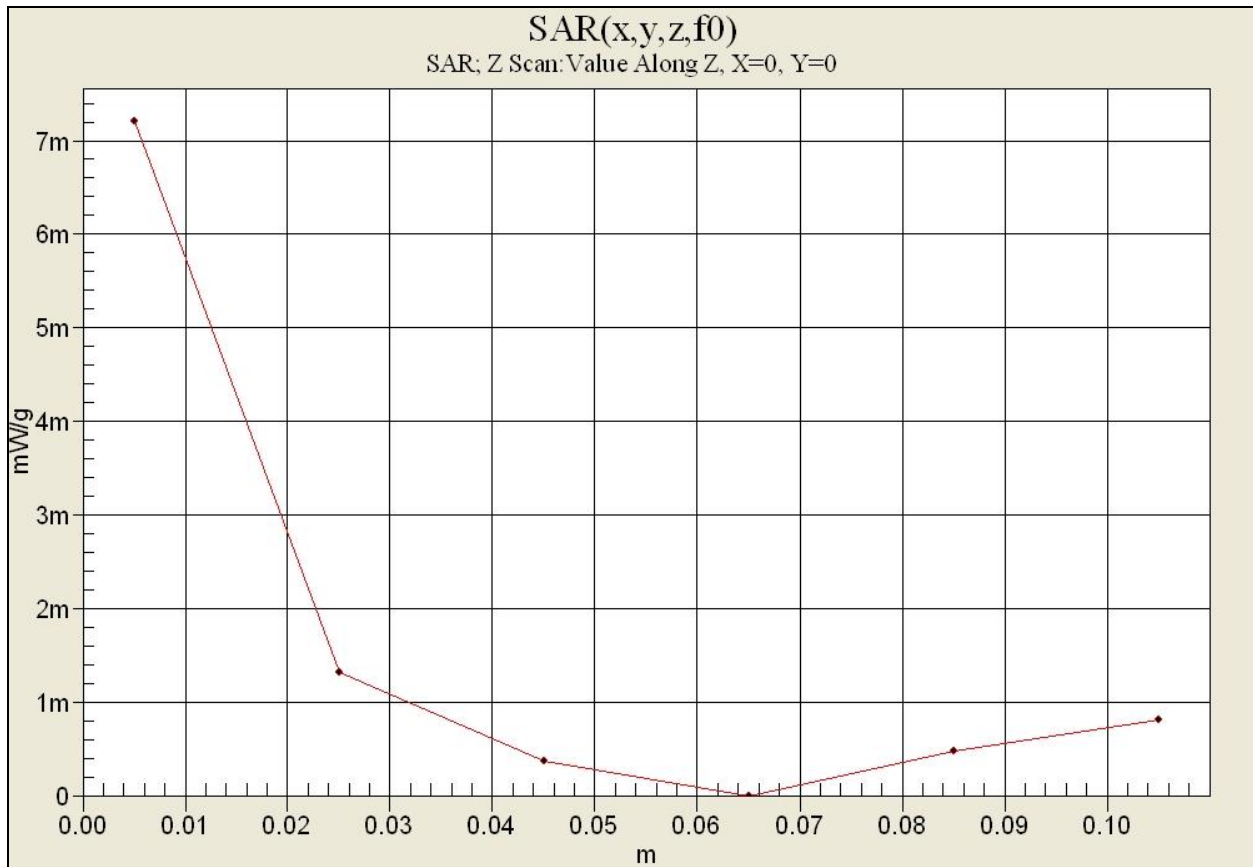
Plot 3. 2440.8MHz Left Head (Z Scan)
