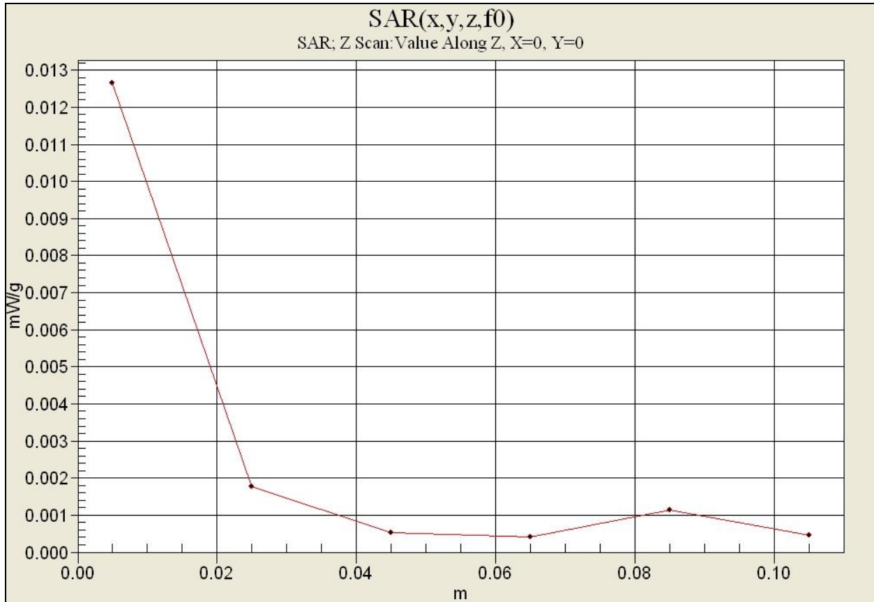
Plot 1. 2401.92MHz Left Head (Z Scan)
