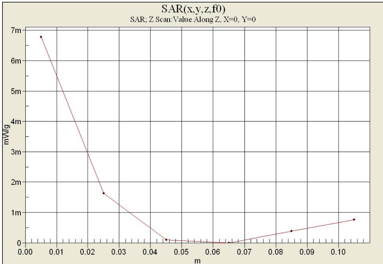
Plot 6. 2479.68MHz Right Head (Z Scan)
