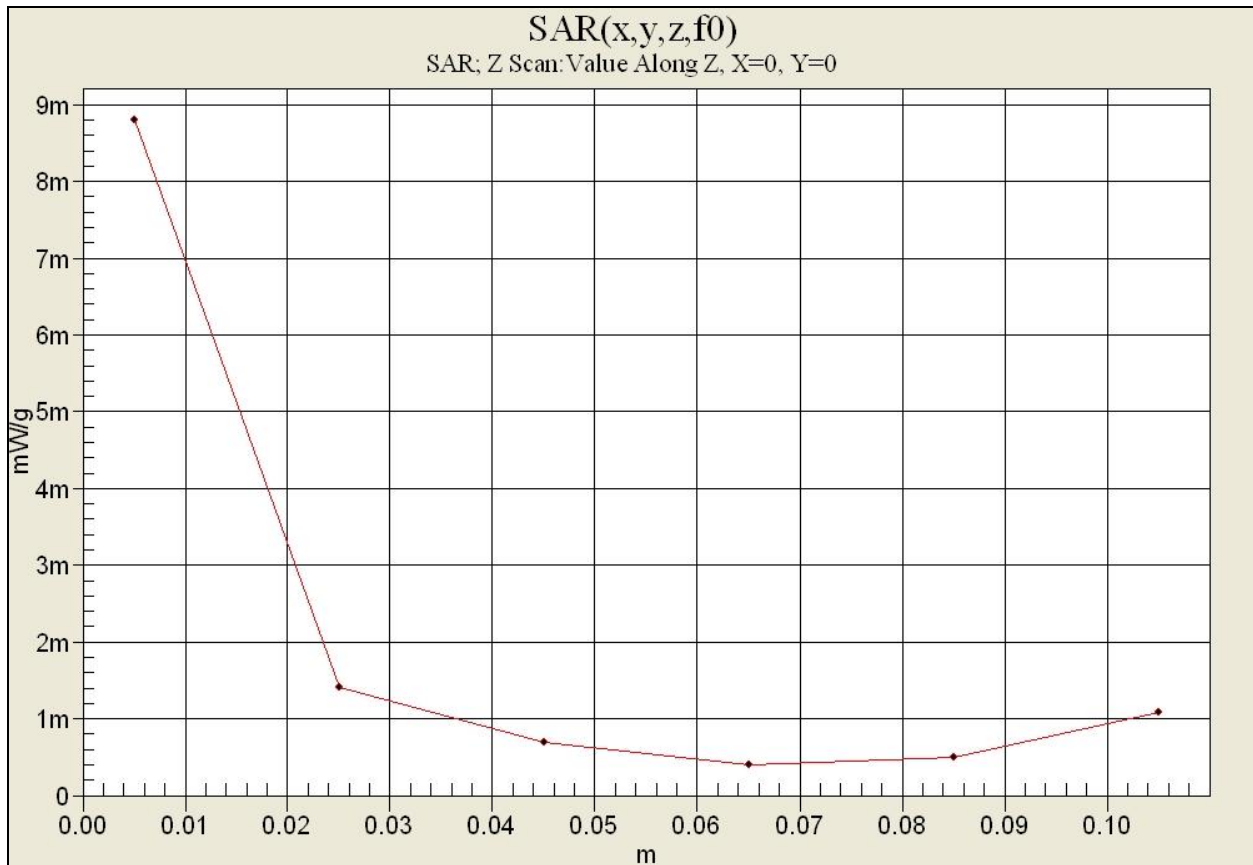
Plot 5. 2479.68MHz Left Head (Z Scan)
