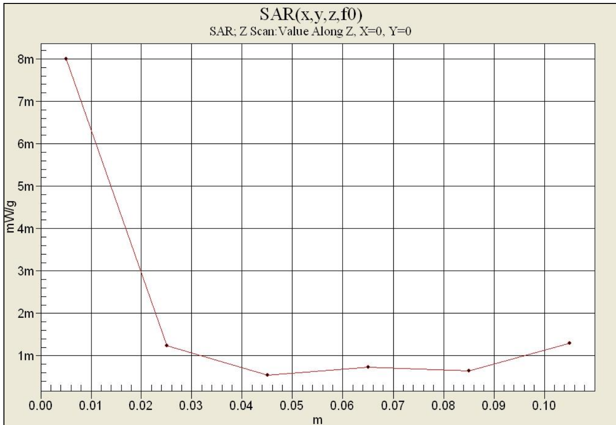
Plot 4. 2440.8MHz Right Head (Z Scan)
