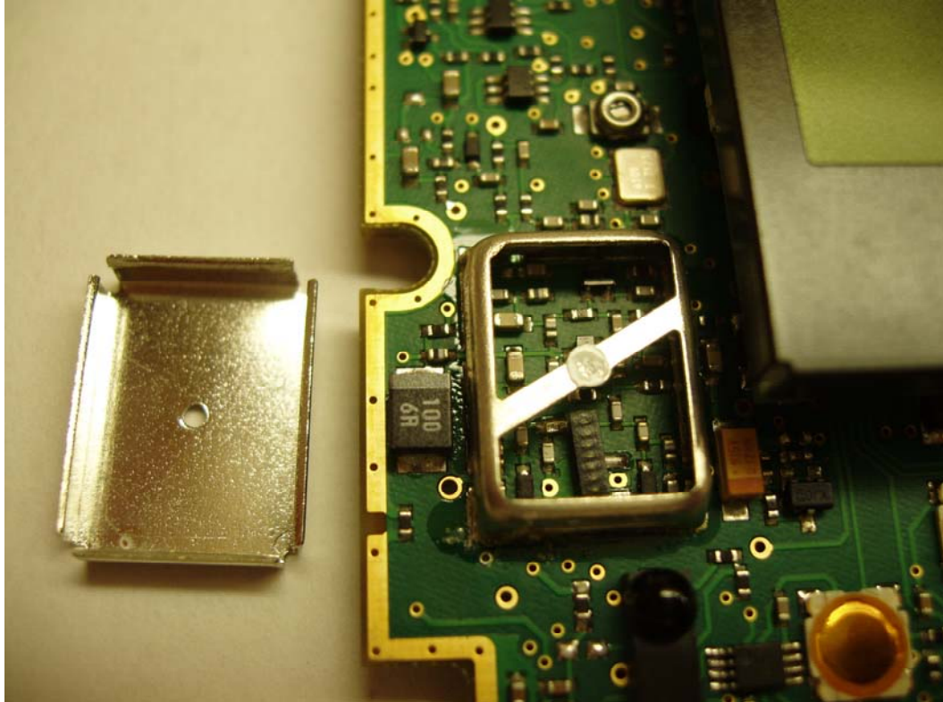
UR1A PCB RF Section
