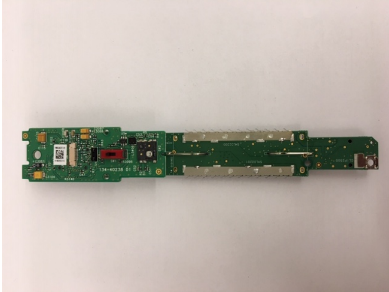
ULXD2 PCB Top
