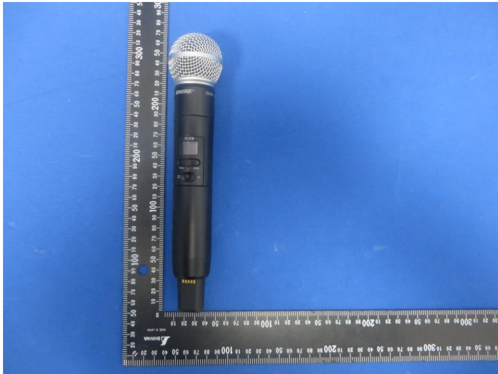
(1) EUT Photo (SLXD2 G58)
