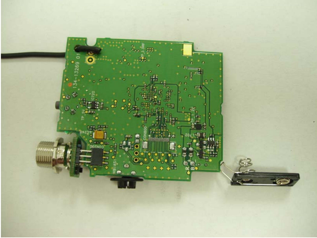
PGXD1 PCB Bottom
