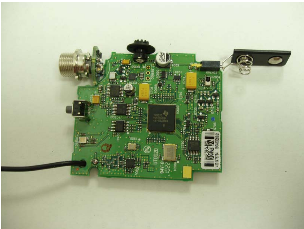
PGXD1 PCB Top
