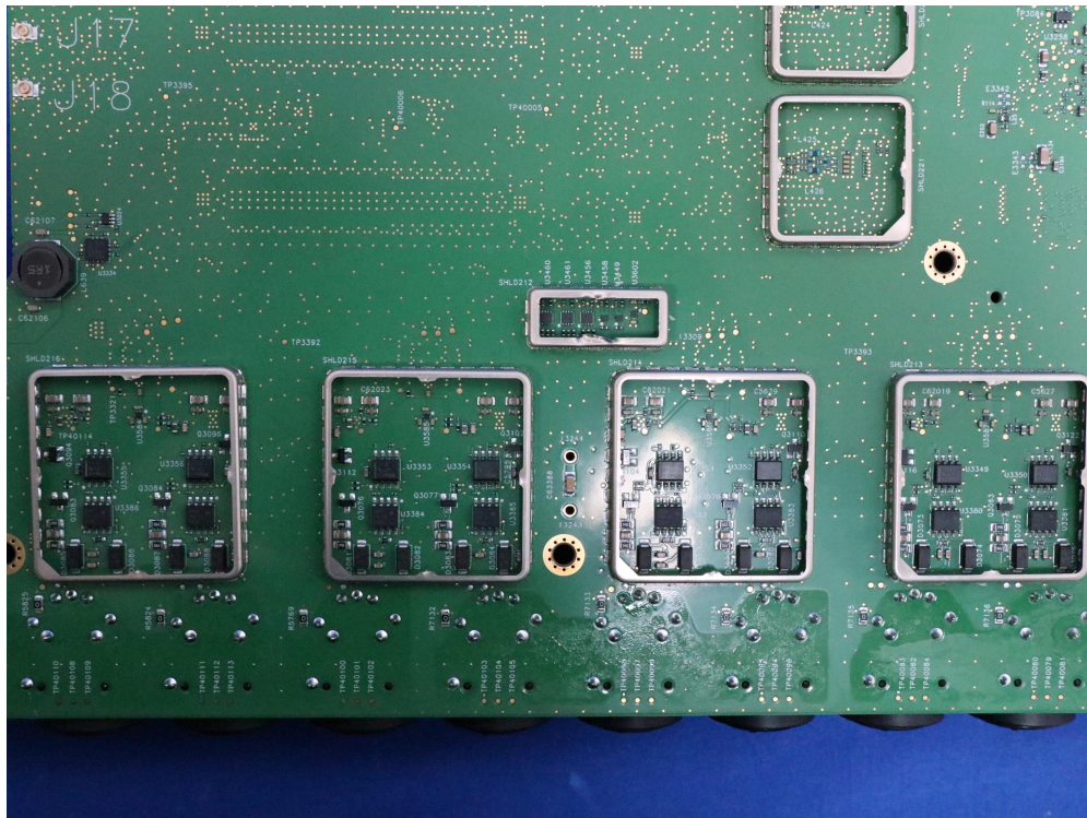
(48) EUT Photo
