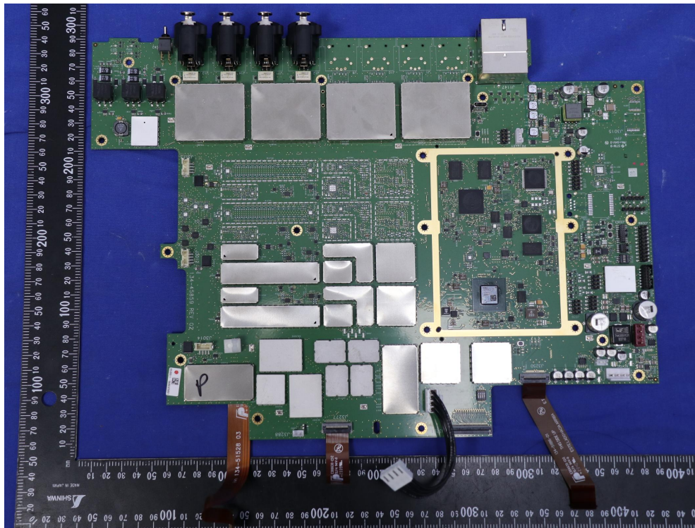
(30) EUT Photo
