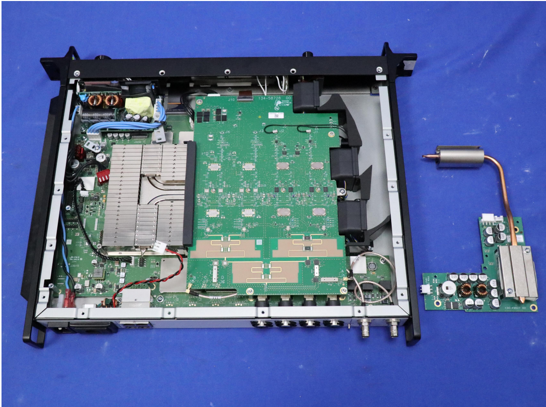
(9) EUT Photo
