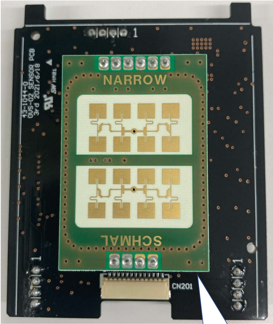
RADIO MODULE
