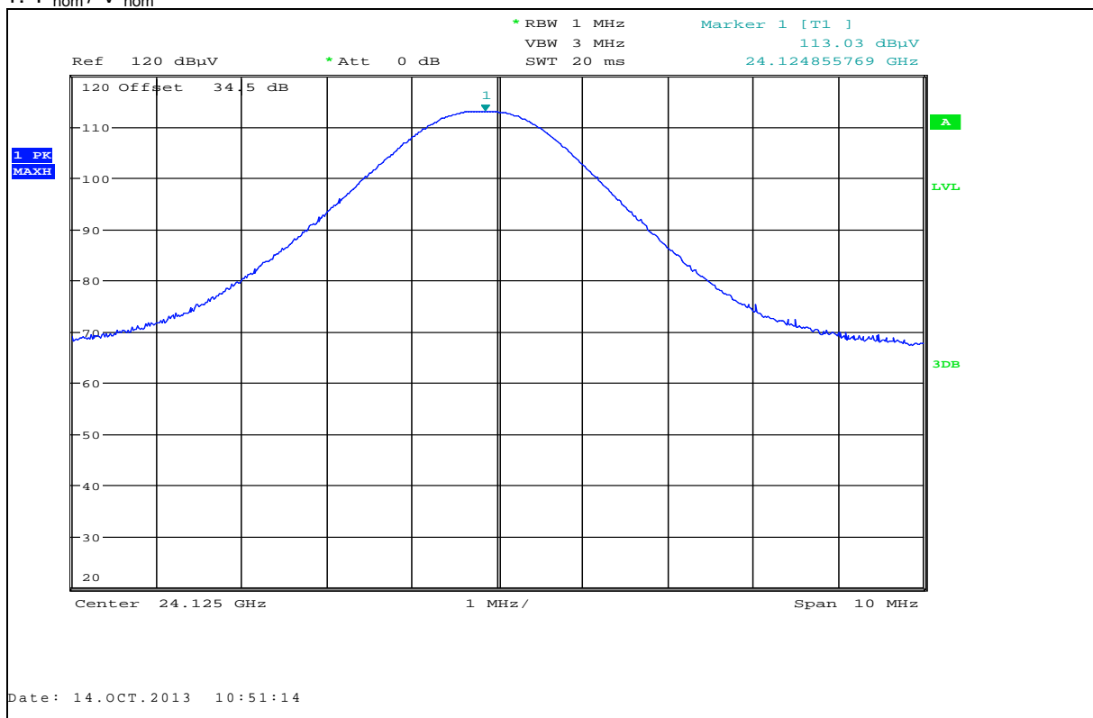
Plot 1: T_{nom} / V_{nom}
