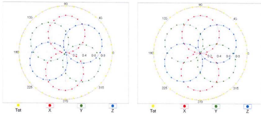
f=1800 MHz,R22
