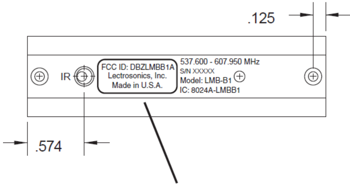
Label location - actual size
