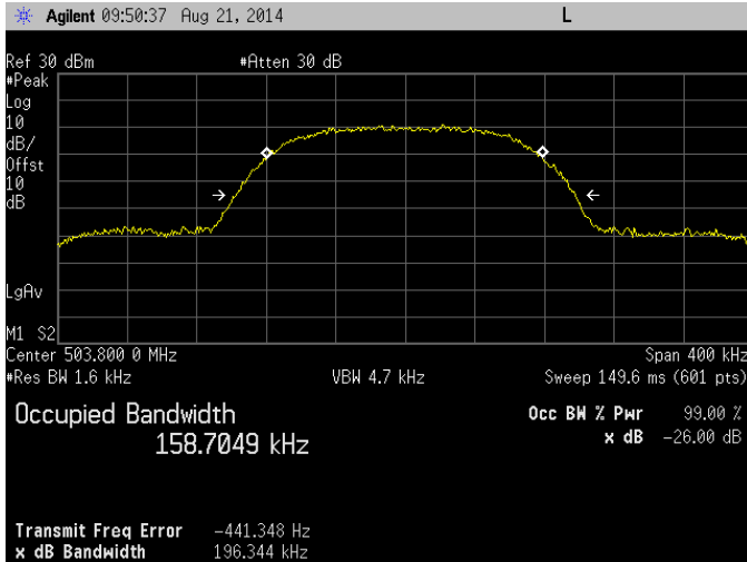
503.800 MHz OBW
