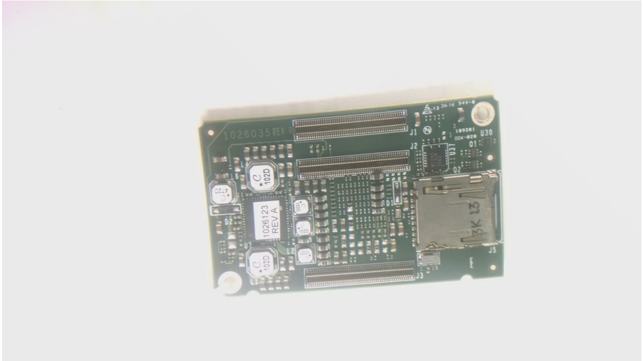
Bottom View of the SOM containing the TI WL1837 WLAN chipset
