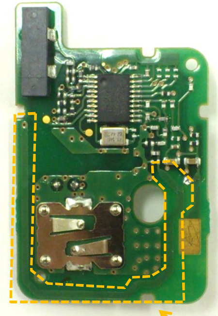
Antenna
