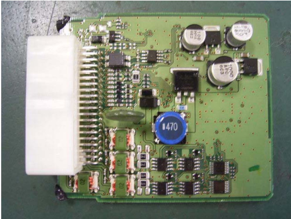
PCB Top
