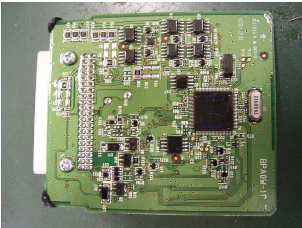
PCB Bottom
