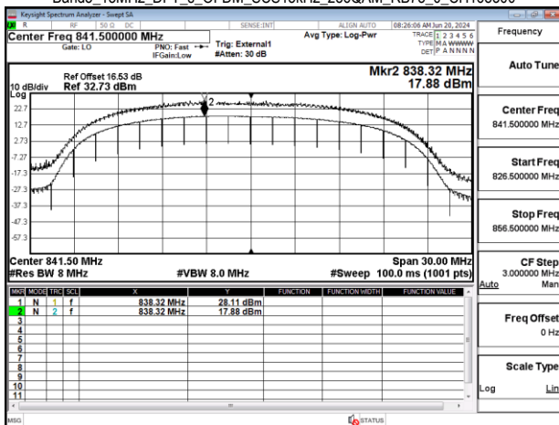
Band5 15MHz DFT s OFDM SCS15kHz 256QAM RB75_0 CH168300
