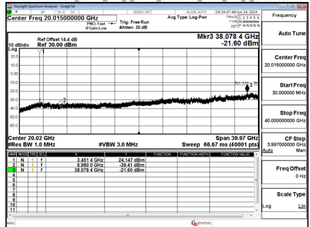
Band77-Part27_80MHz_DFT_s_OFDM_SCS30kHz_BPSK_RB1_1_CH632668
