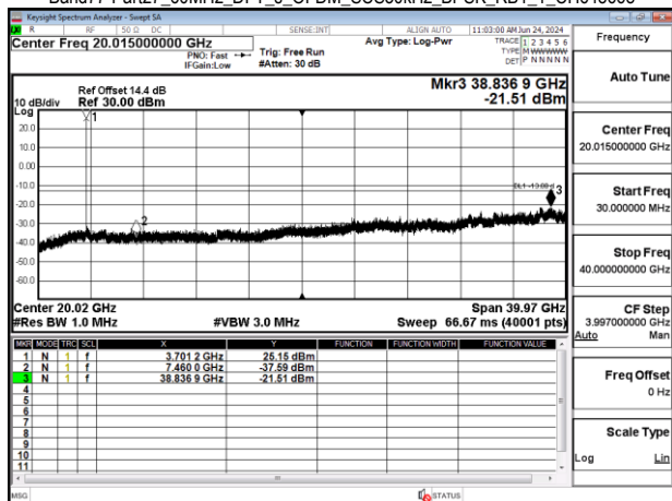
Band77-Part27_60MHz_DFT_s_OFDM_SCS30kHz_BPSK_RB1_1_CH648668
