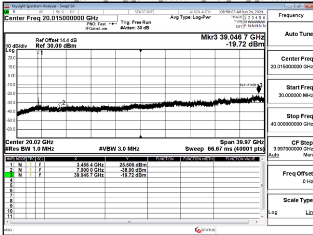
Band77-Part27_90MHz_DFT_s_OFDM_SCS30kHz_BPSK_RB1_1_CH633666
