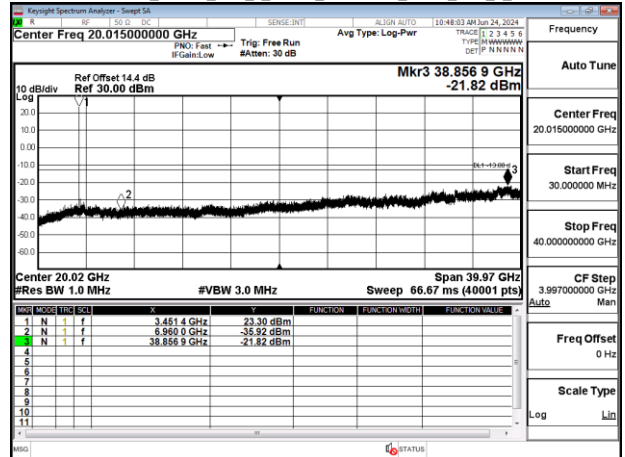
Band77-Part27_60MHz_DFT_s_OFDM_SCS30kHz_BPSK_RB1_1_CH632000
