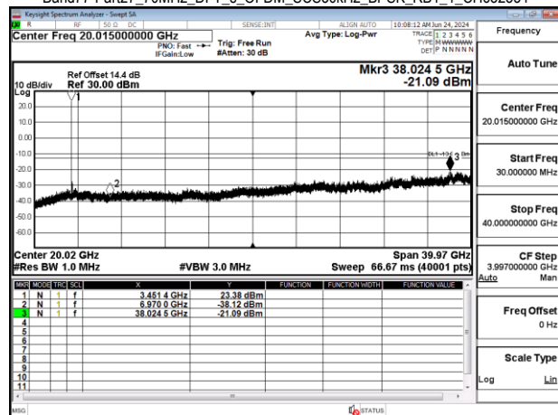
Band77-Part27_70MHz_DFT_s_OFDM_SCS30kHz_BPSK_RB1_1_CH632334
