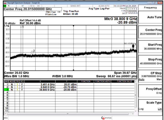
Band77-Part27_40MHz_DFT_s_OFDM_SCS30kHz_BPSK_RB1_1_CH631334
