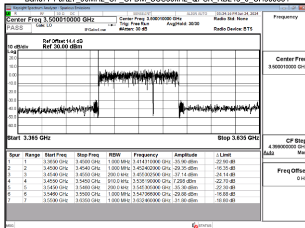
Band77-Part27_90MHz_CP_OFDM_SCS30kHz_QPSK_RB245_0_CH633334
