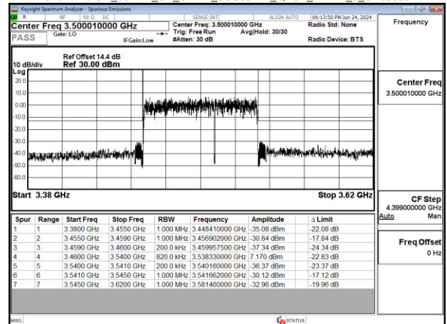
Band77-Part27_80MHz_CP_OFDM_SCS30kHz_QPSK_RB217_0_CH633334
