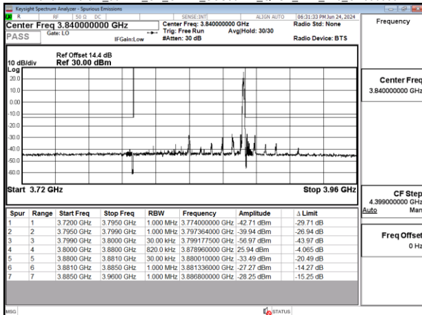
Band77-Part27_80MHz_CP_OFDM_SCS30kHz_QPSK_RB1_216_CH656000
