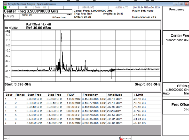
Band77-Part27_70MHz_CP_OFDM_SCS30kHz_QPSK_RB1_0_CH633334
