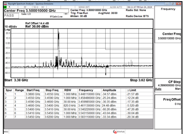
Band77-Part27_80MHz_CP_OFDM_SCS30kHz_QPSK_RB1_0_CH633334
