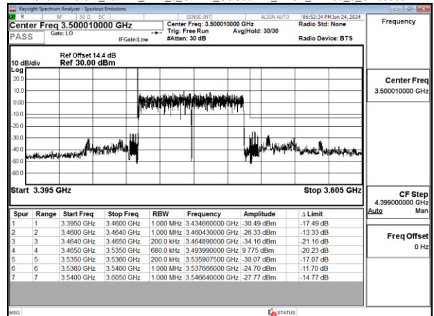
Band77-Part27_70MHz_DFT_s_OFDM_SCS30kHz_BPSK_RB180_0_CH633334
