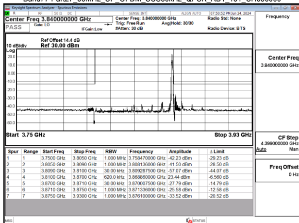
Band77-Part27_60MHz_CP_OFDM_SCS30kHz_QPSK_RB1_161_CH656000
