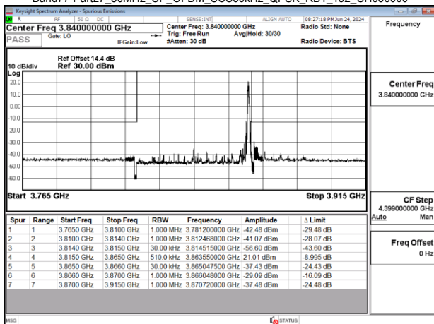
Band77-Part27_50MHz_CP_OFDM_SCS30kHz_QPSK_RB1_132_CH656000
