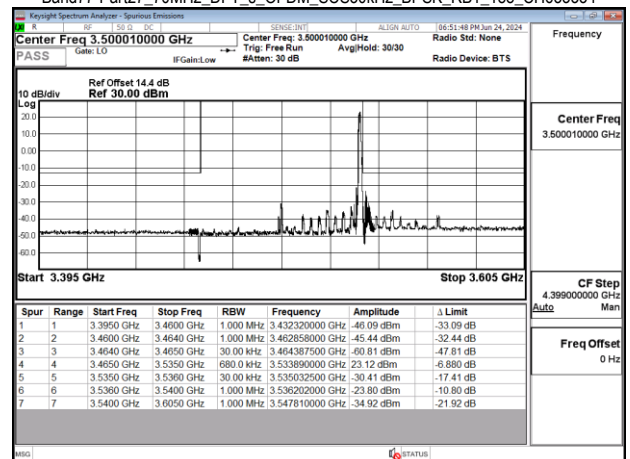
Band77-Part27_70MHz_DFT_s_OFDM_SCS30kHz_BPSK_RB1_188_CH633334
