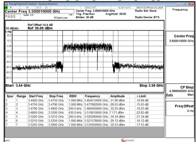
Band77-Part27_40MHz_CP_OFDM_SCS30kHz_QPSK_RB106_0_CH633334
