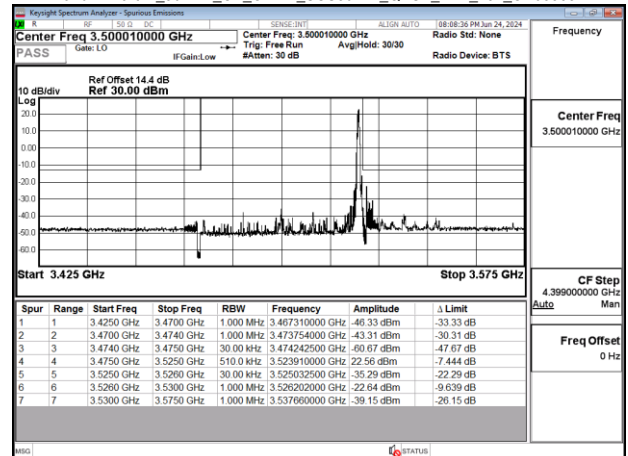
Band77-Part27_50MHz_CP_OFDM_SCS30kHz_QPSK_RB1_132_CH633334
