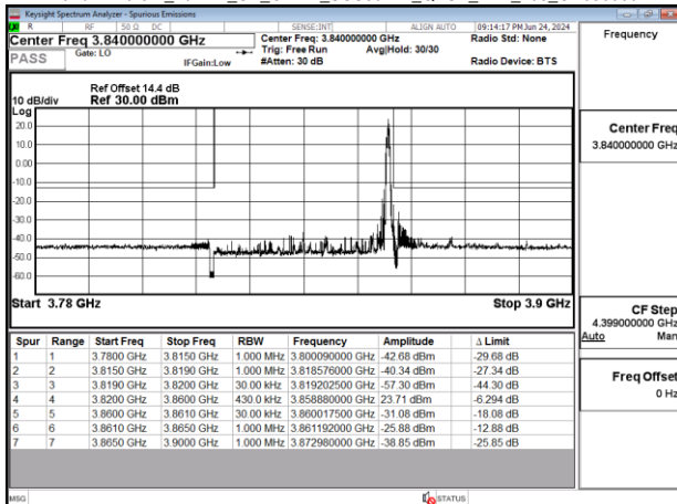
Band77-Part27_40MHz_CP_OFDM_SCS30kHz_QPSK_RB1_105_CH656000
