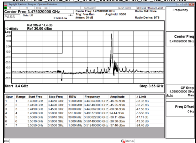
Band77-Part27_50MHz_DFT_s_OFDM_SCS30kHz_BPSK_RB1_132_CH633334
