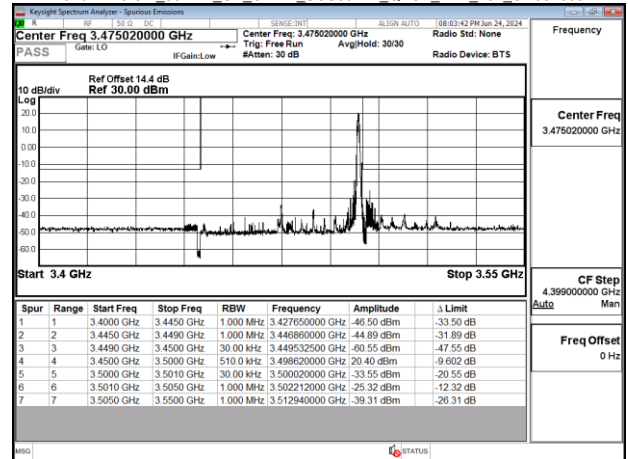
Band77-Part27_50MHz_CP_OFDM_SCS30kHz_QPSK_RB1_132_CH633334
