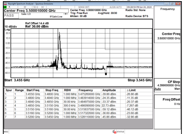
Band77-Part27_30MHz_CP_OFDM_SCS30kHz_QPSK_RB1_0_CH633334
