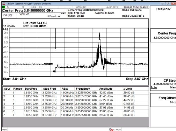
Band77-Part27_20MHz_CP_OFDM_SCS30kHz_QPSK_RB1_50_CH656000
