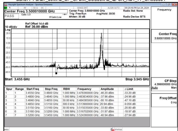
Band77-Part27_30MHz_CP_OFDM_SCS30kHz_QPSK_RB1_77_CH633334
