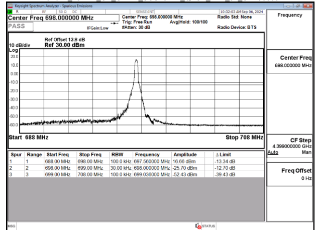
Band71_10MHz_CP_OFDM_SCS15kHz_QPSK_RB52_0_CH138600
