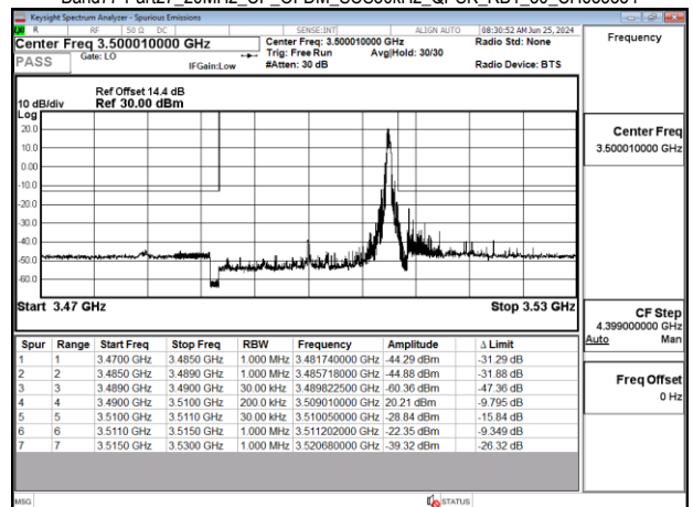
Band77-Part27_20MHz_CP_OFDM_SCS30kHz_QPSK_RB1_50_CH633334
