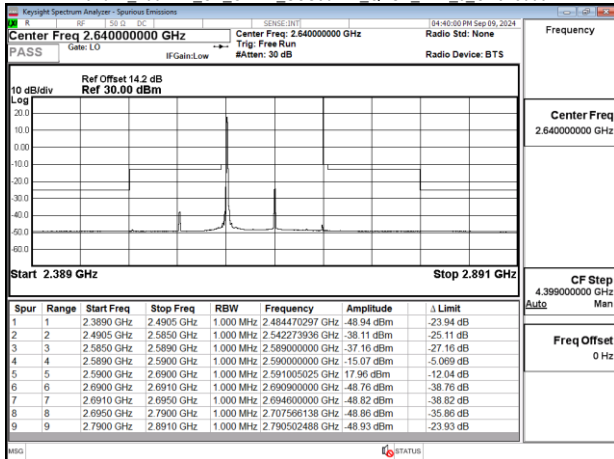
Band41_100MHz_CP_OFDM_SCS30kHz_QPSK_RB1_272_CH509202
