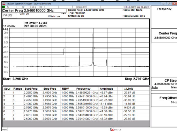
Band41_100MHz_CP_OFDM_SCS30kHz_QPSK_RB1_272_CH509202
