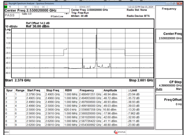
Band41_60MHz_CP_OFDM_SCS30kHz_QPSK_RB1_161_CH518598
