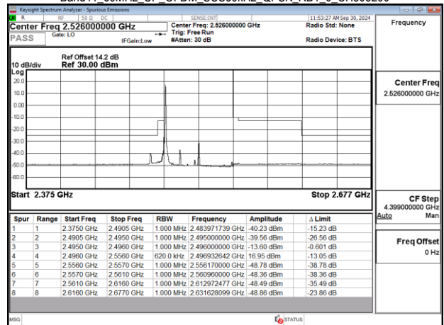
Band41_60MHz_CP_OFDM_SCS30kHz_QPSK_RB1_0_CH506004
