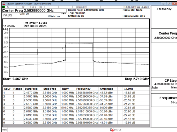
Band41 50MHz CP OFDM_SCS30kHz QPSK RB133 0_CH518598
