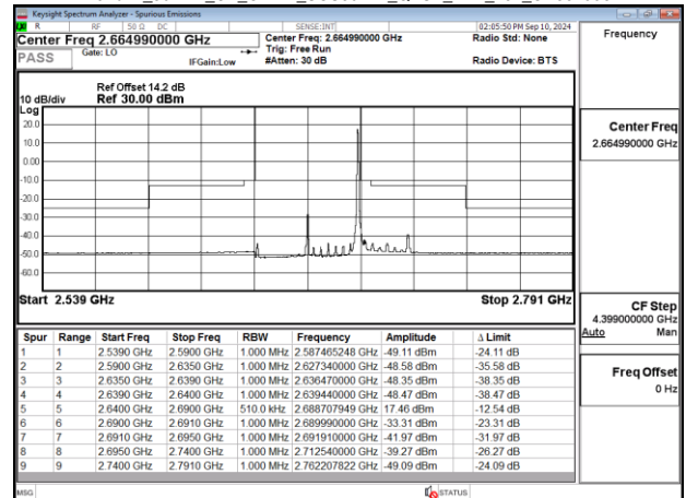
Band41_50MHz_CP_OFDM_SCS30kHz_QPSK_RB1_132_CH532998
