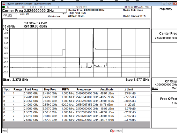
Band41_60MHz_CP_OFDM_SCS30kHz_QPSK_RB1_161_CH505200
