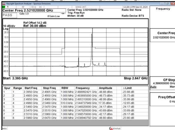
Band41_50MHz_CP_OFDM_SCS30kHz_QPSK_RB1_132_CH504204
