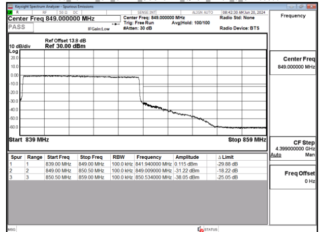
Band5_10MHz_CP_OFDM_SCS15kHz_QPSK_RB52_0_CH168800
