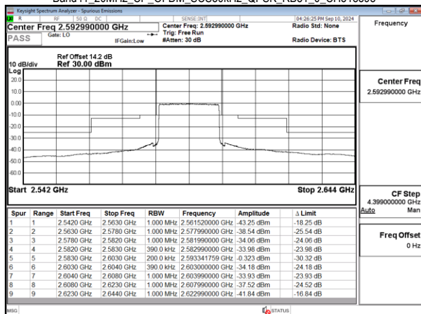
Band41 20MHz CP OFDM_SCS30kHz QPSK RB51_0 CH518598
