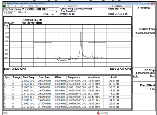
Band41 20MHz_CP_OFDM_SCS30kHz_QPSK_RB1_50_CH535998
