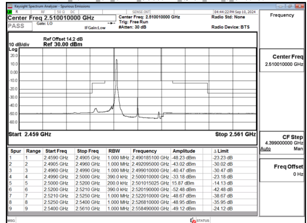
Band41 20MHz CP OFDM SCS30kHz QPSK RB1_0 CH502002
