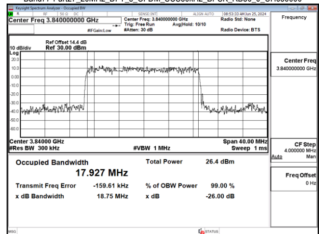
Band77-Part27 20MHz DFT s OFDM_SCS30kHz BPSK_RB50_0 CH656000
