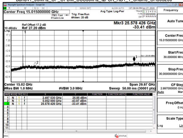
Band41_60MHz_CP_OFDM_SCS30kHz_QPSK_RB1_1_Chain0_CH506004
