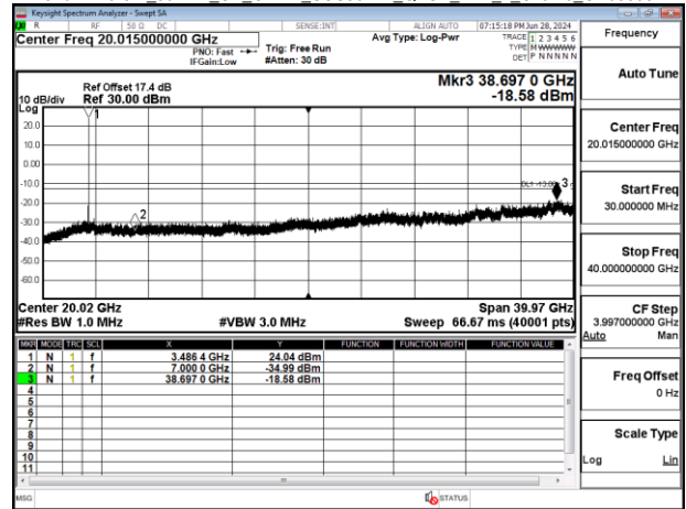
Band77-Part27_30MHz_CP_OFDM_SCS30kHz_QPSK_RB1_1_Chain0_CH635666
