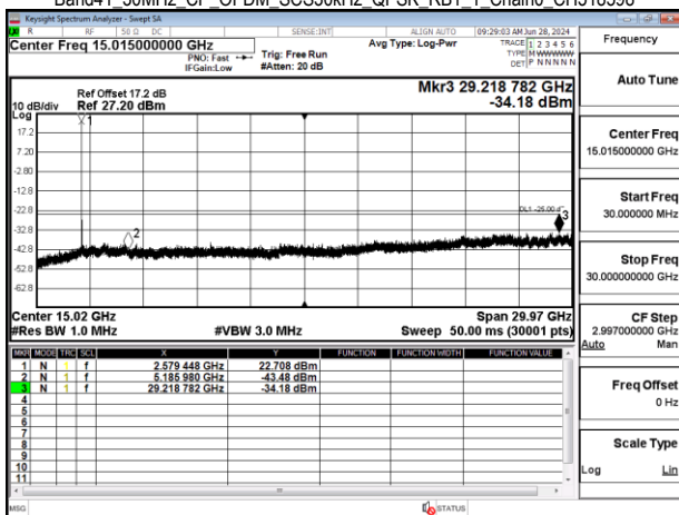
Band41 30MHz CP_OFDM_SCS30kHz_QPSK_RB1_1_Chain0_CH534996
