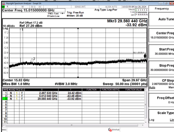
Band41 20MHz CP_OFDM_SCS30kHz_QPSK_RB1_1_Chain0_CH502002
