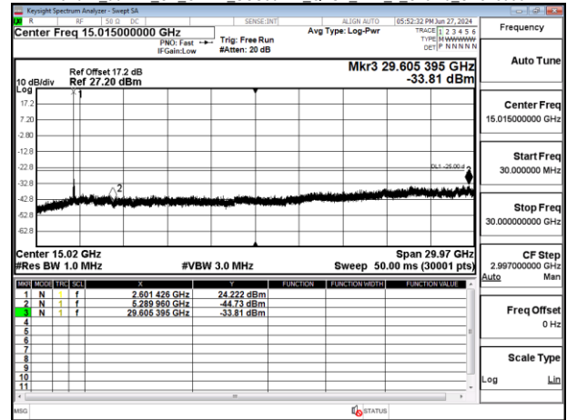
Band41_100MHz_CP_OFDM_SCS30kHz_QPSK_RB1_1_Chain0_CH509202
