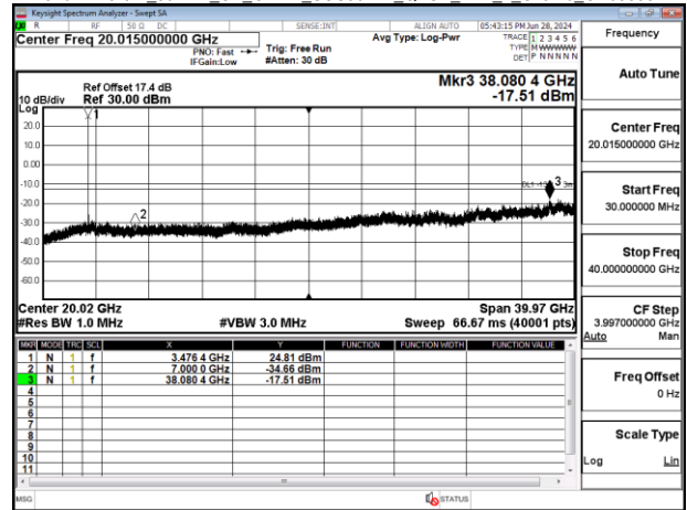
Band77-Part27_50MHz_CP_OFDM_SCS30kHz_QPSK_RB1_1_Chain0_CH635000
