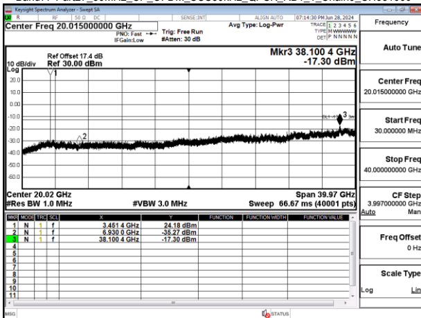
Band77-Part27_30MHz_CP_OFDM_SCS30kHz_QPSK_RB1_1_Chain0_CH631000
