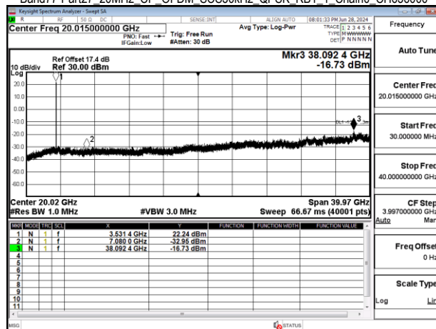
Band77-Part27 20MHz_CP_OFDM_SCS30kHz_QPSK_RB1_1_Chain0_CH647334
