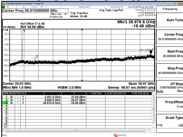
Band77-Part27_40MHz_CP_OFDM_SCS30kHz_QPSK_RB1_1_Chain0_CH631334
