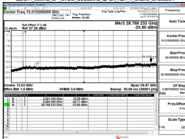
Band41_60MHz_CP_OFDM_SCS30kHz_QPSK_RB1_1_Chain0_CH506004
