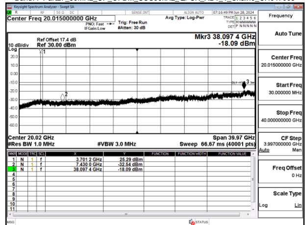
Band77-Part27_30MHz_CP_OFDM_SCS30kHz_QPSK_RB1_1_Chain0_CH647668
