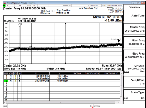
Band77-Part27_50MHz_CP_OFDM_SCS30kHz_QPSK_RB1_1_Chain0_CH648334
