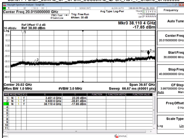
Band77-Part27 20MHz_CP_OFDM_SCS30kHz_QPSK_RB1_1_Chain0_CH630668
