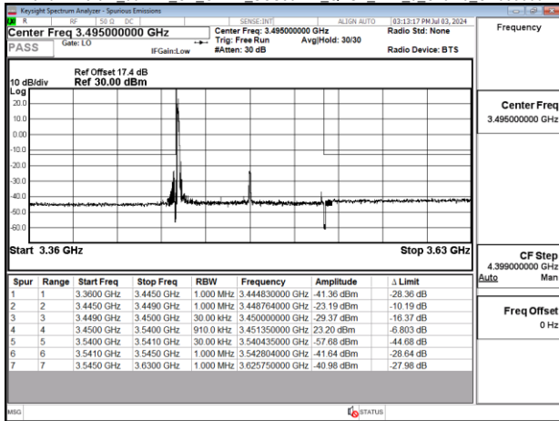
Band77-Part27_90MHz_CP_OFDM_SCS30kHz_QPSK_RB1_0_Chain0_CH633334
