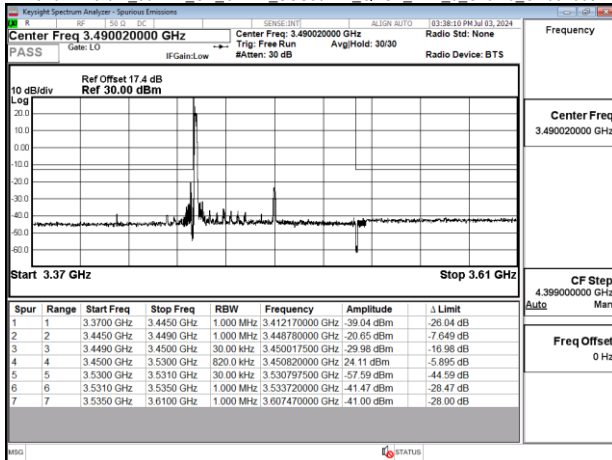
Band77-Part27_80MHz_CP_OFDM_SCS30kHz_QPSK_RB1_0_Chain0_CH633334
