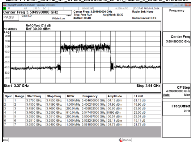
Band77-Part27_90MHz_CP_OFDM_SCS30kHz_QPSK_RB245_0_Chain0_CH633666
