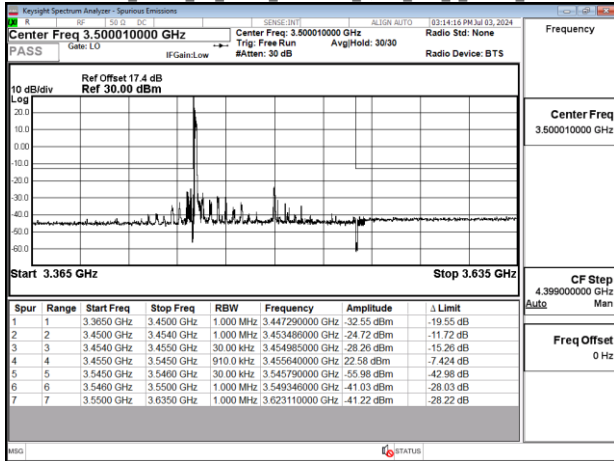
Band77-Part27_90MHz_CP_OFDM_SCS30kHz_QPSK_RB1_0_Chain0_CH633666
