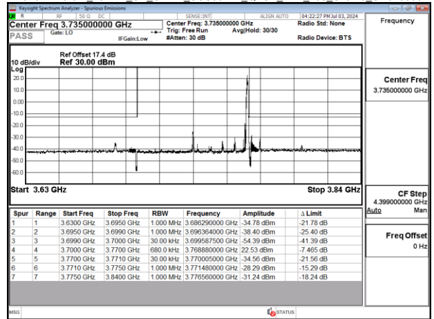
Band77-Part27_70MHz_CP_OFDM_SCS30kHz_QPSK_RB1_188_Chain0_CH656000
