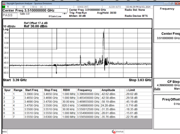
Band77-Part27_80MHz_CP_OFDM_SCS30kHz_QPSK_RB1_216_Chain0_CH634000
