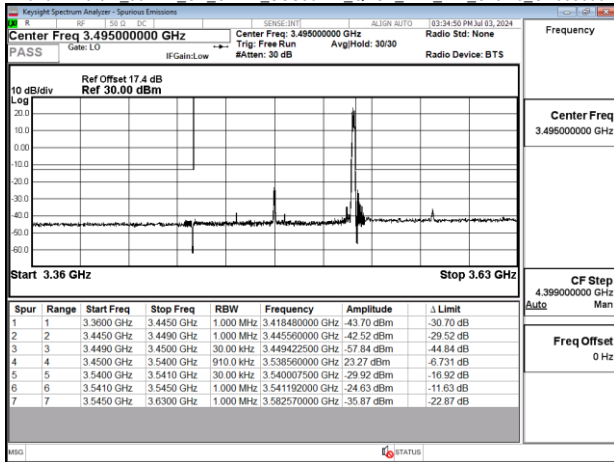
Band77-Part27_90MHz_CP_OFDM_SCS30kHz_QPSK_RB1_244_Chain0_CH633334
