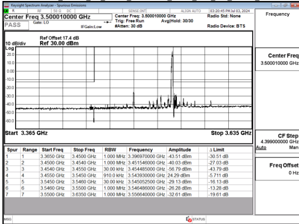
Band77-Part27_90MHz_CP_OFDM_SCS30kHz_QPSK_RB1_244_Chain0_CH633666
