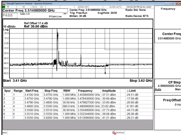
Band77-Part27_70MHz_CP_OFDM_SCS30kHz_QPSK_RB1_0_Chain0_CH634332
