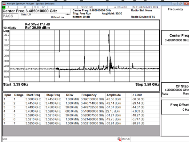
Band77-Part27_70MHz_CP_OFDM_SCS30kHz_QPSK_RB1_188_Chain0_CH633334
