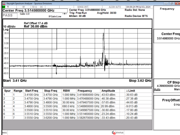
Band77-Part27_70MHz_CP_OFDM_SCS30kHz_QPSK_RB1_188_Chain0_CH634332
