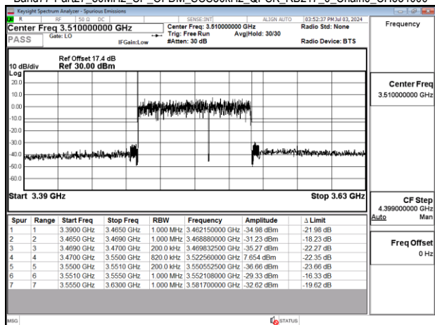
Band77-Part27_80MHz_CP_OFDM_SCS30kHz_QPSK_RB217_0_Chain0_CH634000
