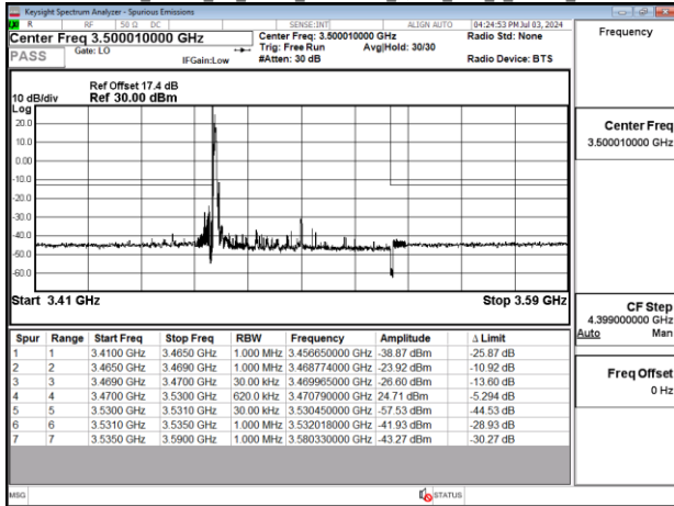
Band77-Part27_60MHz_CP_OFDM_SCS30kHz_QPSK_RB1_0_Chain0_CH634666
