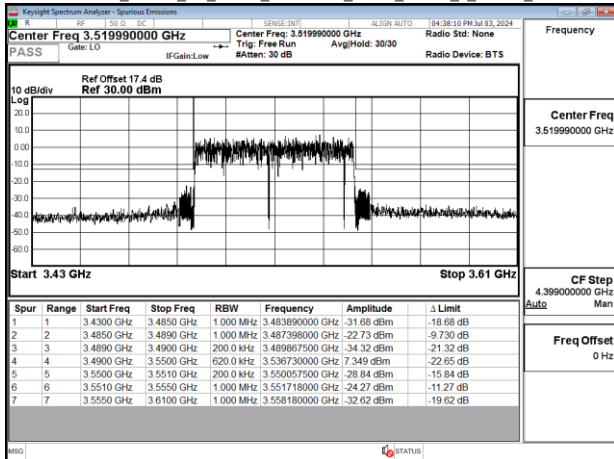
Band77-Part27_60MHz_CP_OFDM_SCS30kHz_QPSK_RB162_0_Chain0_CH634666
