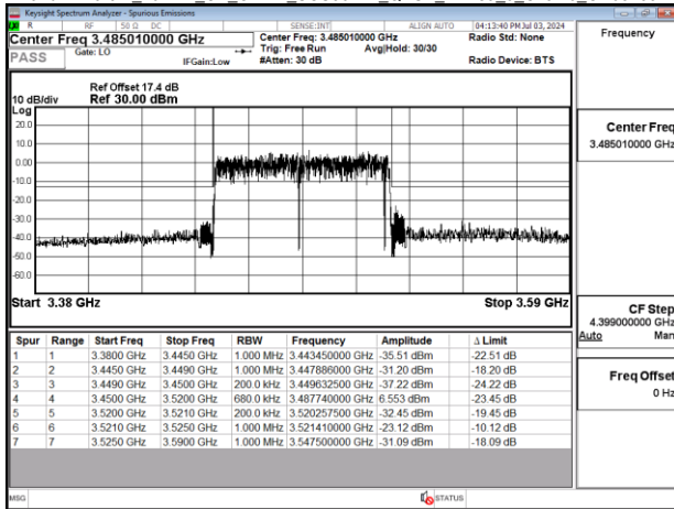
Band77-Part27_70MHz_CP_OFDM_SCS30kHz_QPSK_RB189_0_Chain0_CH633334
