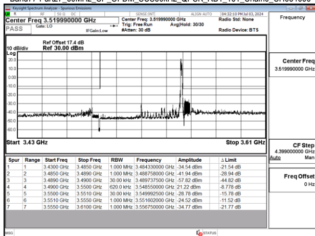
Band77-Part27_60MHz_CP_OFDM_SCS30kHz_QPSK_RB1_161_Chain0_CH634666
