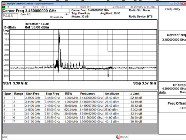
Band77-Part27_60MHz_CP_OFDM_SCS30kHz_QPSK_RB1_0_Chain0_CH633334
