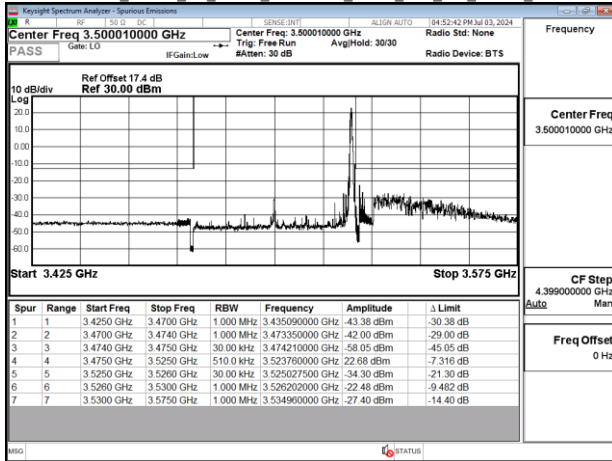
Band77-Part27_50MHz_CP_OFDM_SCS30kHz_QPSK_RB1_132_Chain0_CH635000
