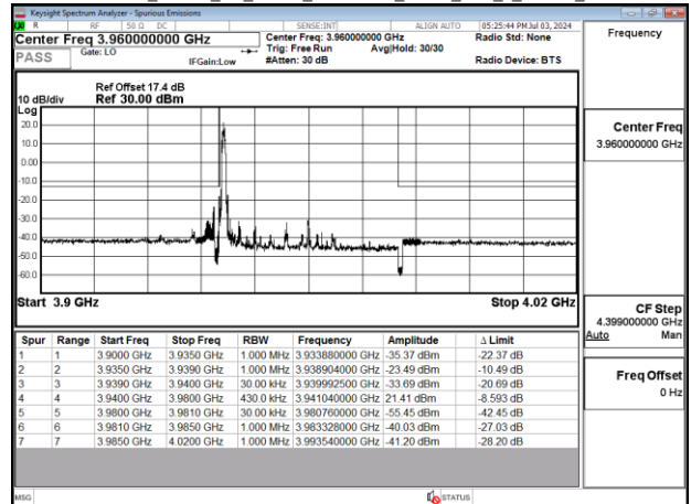
Band77-Part27 40MHz CP OFDM SCS30kHz QPSK RB1_0 Chain0 CH664000
