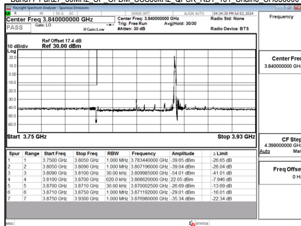
Band77-Part27_60MHz_CP_OFDM_SCS30kHz_QPSK_RB1_161_Chain0_CH633332
