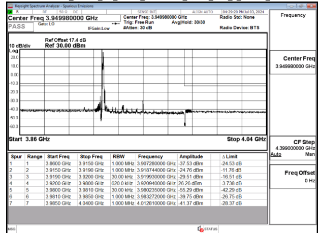
Band77-Part27_60MHz_CP_OFDM_SCS30kHz_QPSK_RB1_0_Chain0_CH663332
