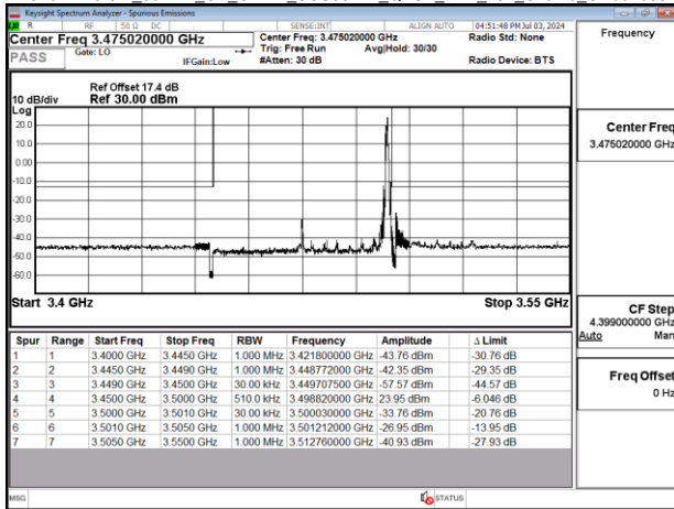
Band77-Part27_50MHz_CP_OFDM_SCS30kHz_QPSK_RB1_132_Chain0_CH633334
