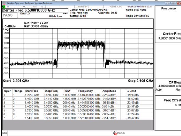
Band77-Part27_70MHz_CP_OFDM_SCS30kHz_QPSK_RB189_0_Chain0_CH634332
