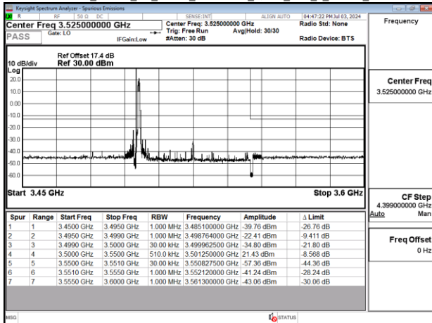
Band77-Part27_50MHz_CP_OFDM_SCS30kHz_QPSK_RB1_0_Chain0_CH635000
