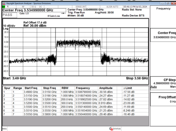
Band77-Part27_30MHz_CP_OFDM_SCS30kHz_QPSK_RB78_0_Chain0_CH635666
