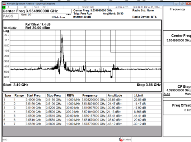
Band77-Part27_30MHz_CP_OFDM_SCS30kHz_QPSK_RB1_0_Chain0_CH635666
