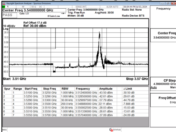
Band77-Part27_20MHz_CP_OFDM_SCS30kHz_QPSK_RB1_50_Chain0_CH636000
