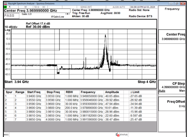
Band77-Part27_20MHz_CP_OFDM_SCS30kHz_QPSK_RB1_50_Chain0_CH664666
