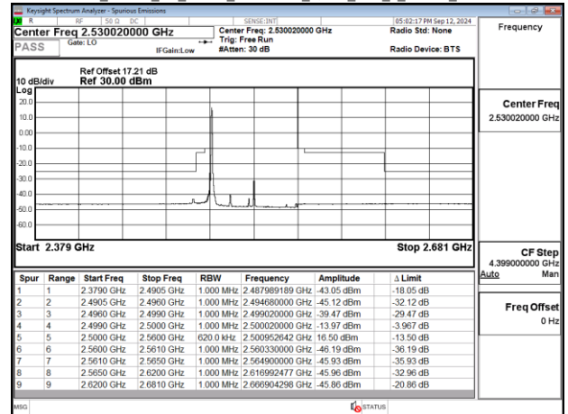
Band41_60MHz_CP_OFDM_SCS30kHz_QPSK_RB1_0_Chain0_CH506004
