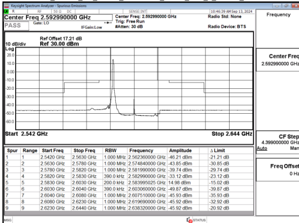
Band41 20MHz CP OFDM SCS30kHz QPSK RB1_0 Chain0_CH518598
