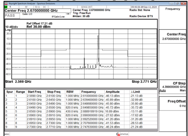
Band41 40MHz CP OFDM SCS30kHz QPSK RB1_105 Chain0_CH534000
