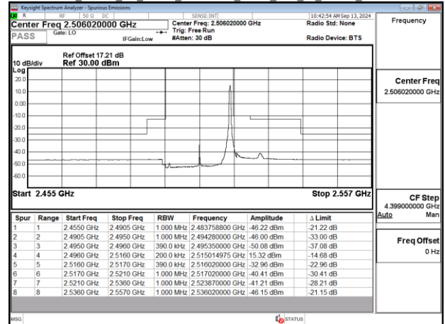
Band41 20MHz CP OFDM SCS30kHz QPSK RB1_50 Chain0_CH502002
