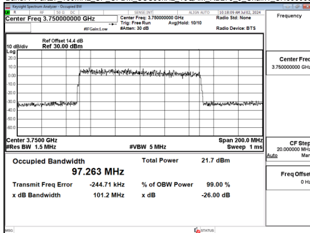
Band77-Part27 100MHz CP OFDM SCS30kHz 16QAM RB273 0 Chain1 CH650000
