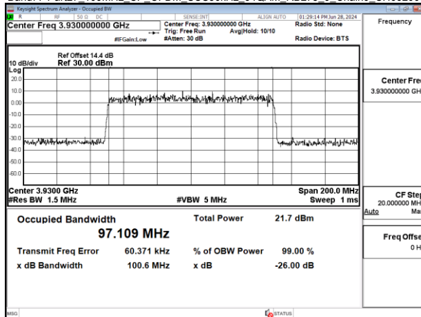
Band77-Part27 100MHz CP OFDM SCS30kHz 64QAM RB273 0 Chain0 CH662000
