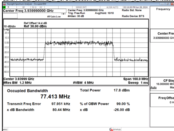
Band77-Par127 80MHz CP OFDM SCS30kHz 256QAM RB217 0 Chain1 CH632668
