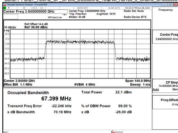
Band77-Part27 70MHz CP OFDM SCS30kHz 16QAM RB189 0 Chain0 CH656000
