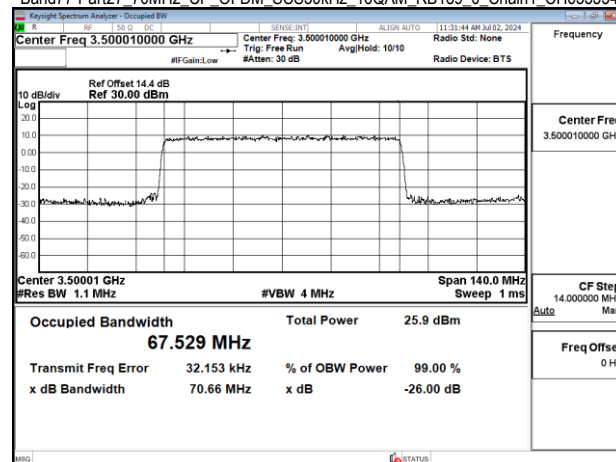
Band77-Part27 70MHz CP OFDM SCS30kHz 16QAM RB189 0 Chain1 CH633334
