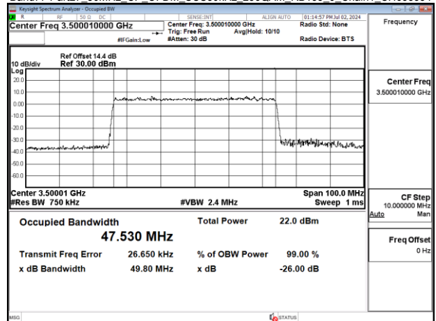
Band77-Part27 50MHz CP OFDM SCS30kHz 256QAM RB133 0 Chain1 CH633334
