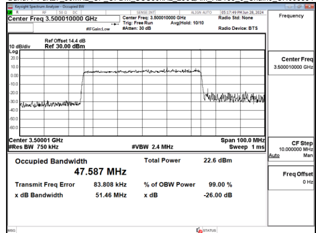
Band77-Part27 50MHz CP OFDM SCS30kHz 256QAM RB133_0 Chain0_CH633334
