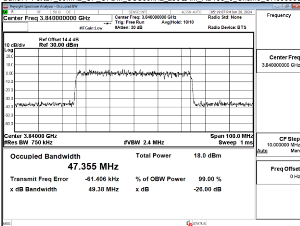
Band77-Part27 50MHz CP OFDM SCS30kHz 256QAM RB133 0 Chain0 CH656000
