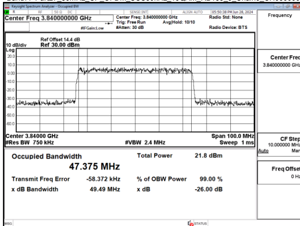
Band77-Part27 50MHz CP OFDM SCS30kHz 16QAM RB133 0 Chain0_CH656000
