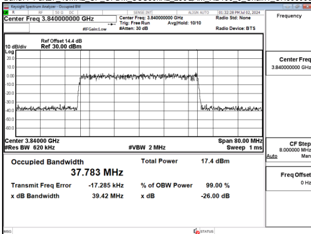
Band77-Part27 40MHz CP OFDM SCS30kHz 256QAM RB106 0 Chain1 CH656000
