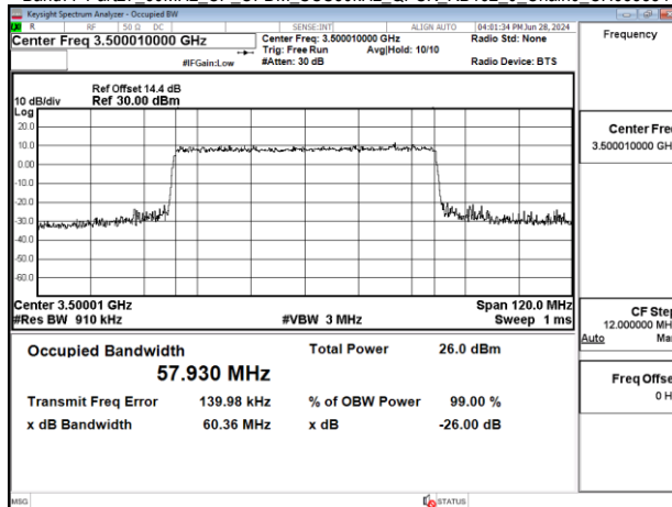
Band77-Part27 60MHz CP OFDM SCS30kHz QPSK RB162 0 Chain0 CH633334
