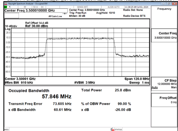
Band77-Part27_60MHz_CP_OFDM_SCS30kHz_QPSK_RB162_0_Chain1_CH633334
