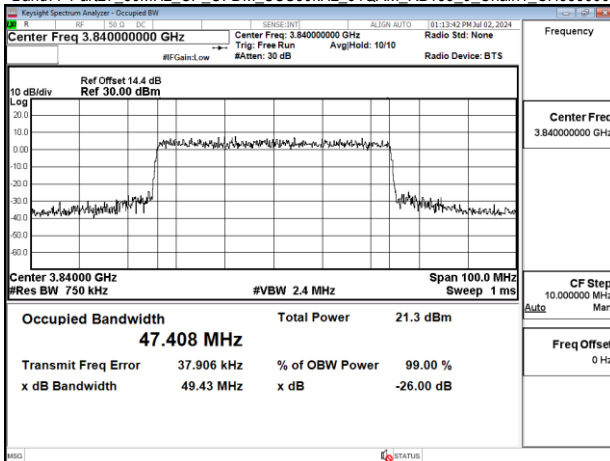
Band77-Part27 50MHz CP OFDM SCS30kHz 64QAM RB133_0 Chain1_CH656000
