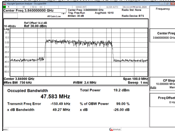
Band77-Part27 50MHz CP OFDM SCS30kHz 16QAM RB133 0 Chain1 CH656000
